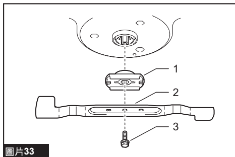
► 1. 刀片支撐座 2. 修剪機刀片 3. 螺栓
