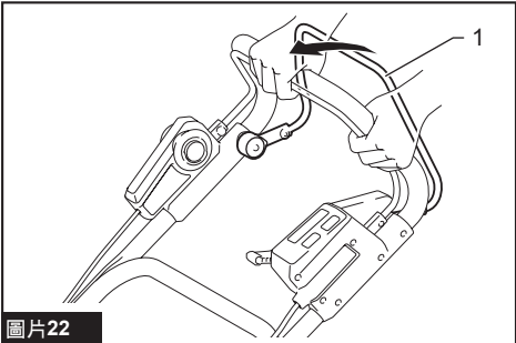
► 1. 驅動桿
