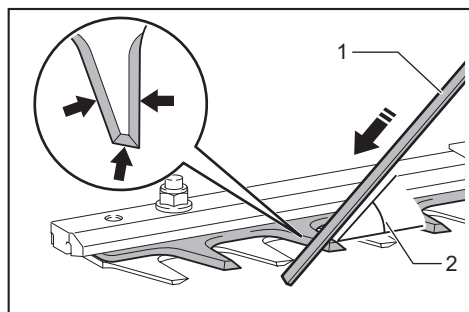
► (1) 銼刀 (2) 45^\circ
