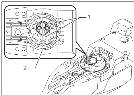
► 1. 開孔 2. 對齊線
