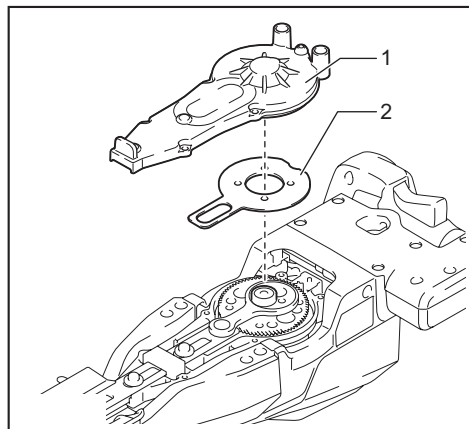
► 1. Cover 2. Plate
