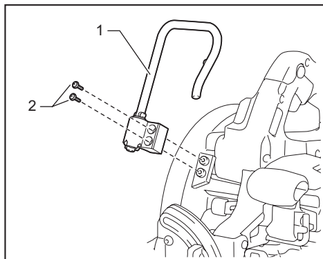
► 1. 鉤環 2. 螺絲
