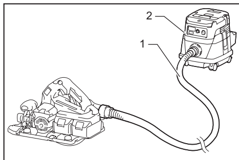
► 1. 軟管 2. 吸塵器
