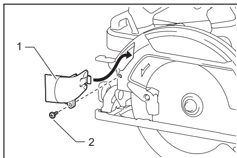
► 1. 集塵噴嘴 2. 螺絲
