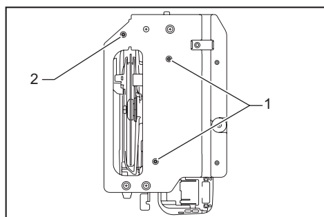
► 1. 0^\circ 角度調整螺絲 2. 45^\circ 角度調整螺絲
