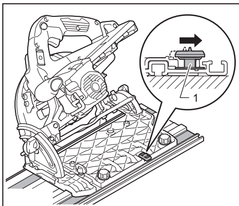
► 1. 滑桿
