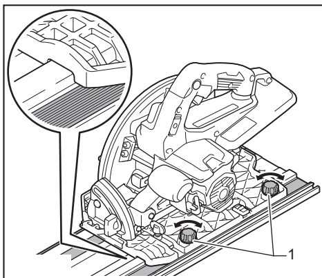
► 1. 調整螺絲
