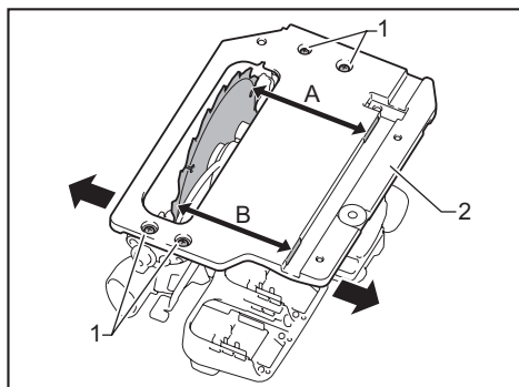
► 1. 螺絲 2. 基座
