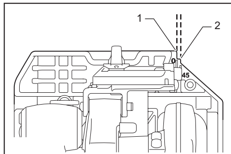
► 1. 切割線 (0° 位置) 2. 切割線 (45° 位置)
