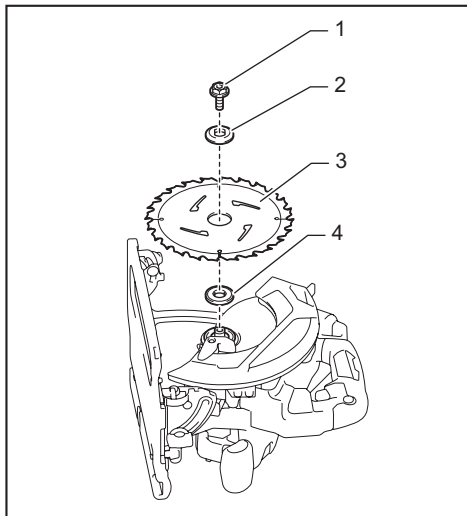
► 1. 六角螺栓 2. 外法蘭 3. 圓鋸機鋸片 4. 內法蘭盤
