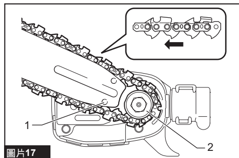
► 1. 開孔 2. 鏈輪
