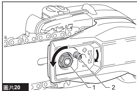
► 1. 固定螺帽 2. 鏈條調整螺絲
