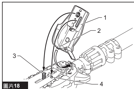
► 1. 鏈輪護蓋 2. 凸起部分 3. 螺栓 4. 插銷
