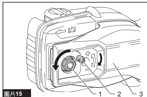
► 1. 固定螺帽 2. 鏈條調整螺絲 3. 鏈輪護蓋
