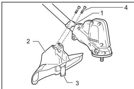
► 1. 固定夾 2. 安全保護裝置 3. 刀具 4. 螺栓
