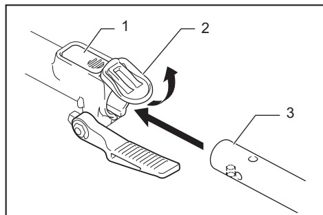
► 1. 鎖定桿 2. 接合處外蓋 3. 連接管
