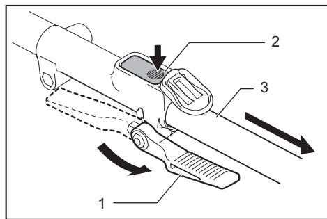
► 1. 固定桿 2. 鎖定桿 3. 連接管
