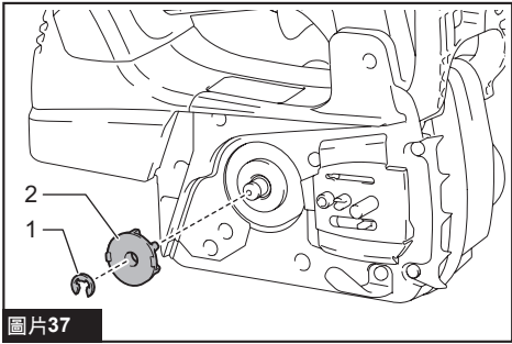
► 1. 鎖定環 2. 鏈輪
