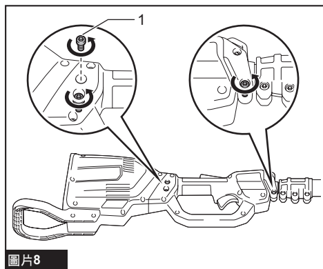
► 1. 螺栓
