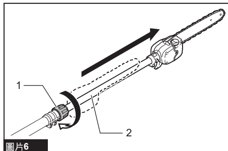
► 1. 鎖定環 2. 管件
