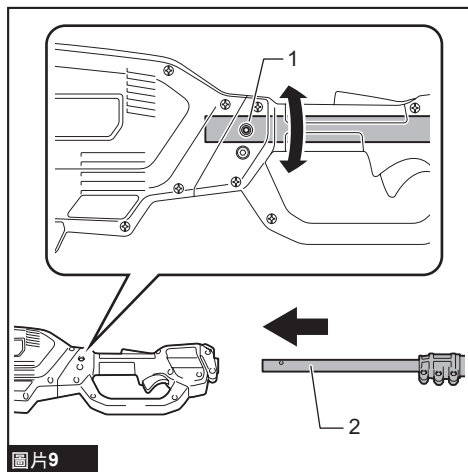
► 1. 開孔 2. 管件
