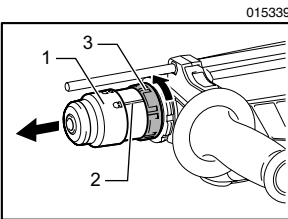
1. SDS-plus 的快换式卡盘 2. 转换套指示线 3. 转换套
