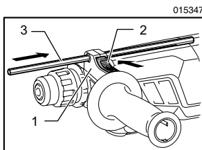
1. 把手基座 2. 锁定按钮 3. 深度规
