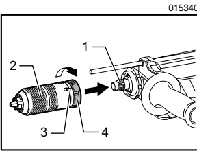
1. 主轴 2. 快换式钻机卡盘 3. 转换套指示线 4. 转换套
