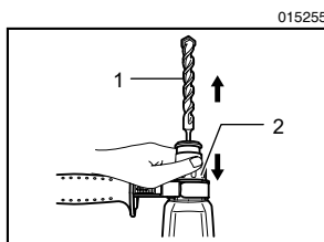
1. 钻头 2. 卡盘壳
