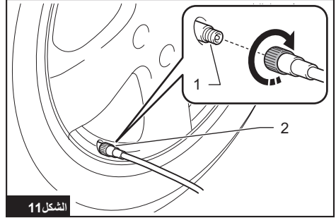
1. ساق الصمام 2. ماسك اللقمة الهوائي
