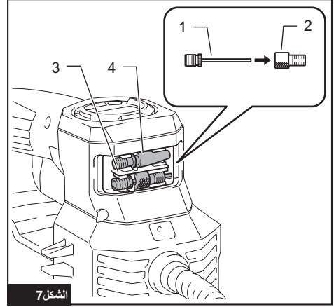
الشكل 7 1. إبرة كرة القدم 2. مهايئ صمام بريسيتا 3. حامل المهايئ 4. المهايئ المدبب
