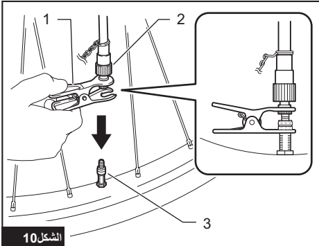
1. مهايئ الصمام الإنجليزي 2. ماسك اللقمة الهوائي 3. ساق الصمام
