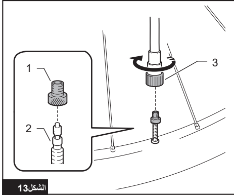
1. مهايئ صمام بريستا 2. ساق الصمام 3. ماسك اللقمة الهوائي
