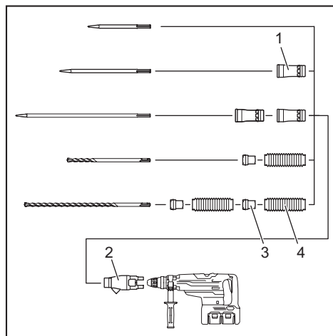
► 1. 防塵蓋板延伸部 2. 防塵蓋板 3. 接頭 4. 伸縮接管
