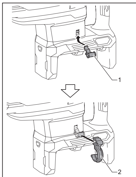
► 1. 固定器接頭 2. 軟管固定器
