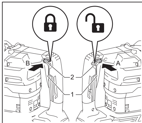
► 1. 開關扳機 2. 扳機鎖定鈕
