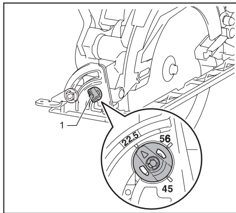
► 1. 主動止動器
