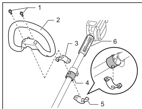
► 1. 內六角螺栓 2. 把手 3. 上方固定夾 4. 減震墊 5. 下方固定夾 6. 墊塊
