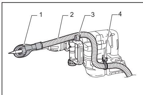
► 1. 防塵蓋板 2. 軟管 3. 軟管固定器 (A/B) 4. 軟管固定器 (C)
