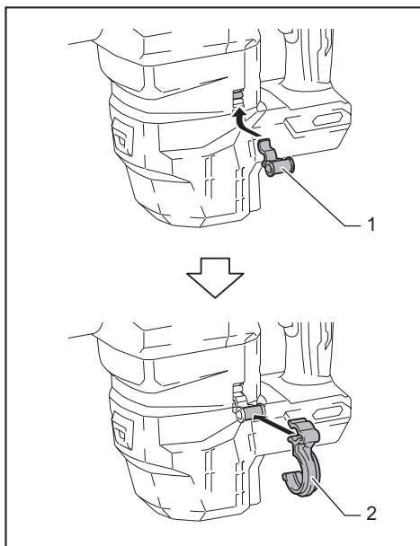
► 1. 固定器接頭 2. 軟管固定器 (C)
