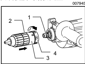
1. 心轴 2. 快换式钻机夹盘 3. 转换套指示线 4. 转换套
