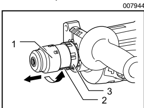
1. SDS-plus 的快换式夹盘 2. 转换套指示线 3. 转换套
