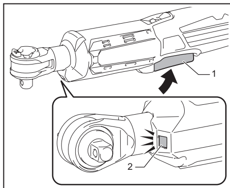
► 1. 開關桿 2. 燈
