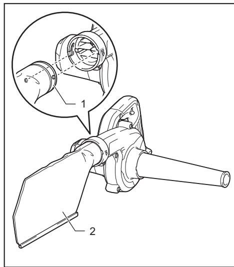
► 1. 接頭 2. 集塵袋
