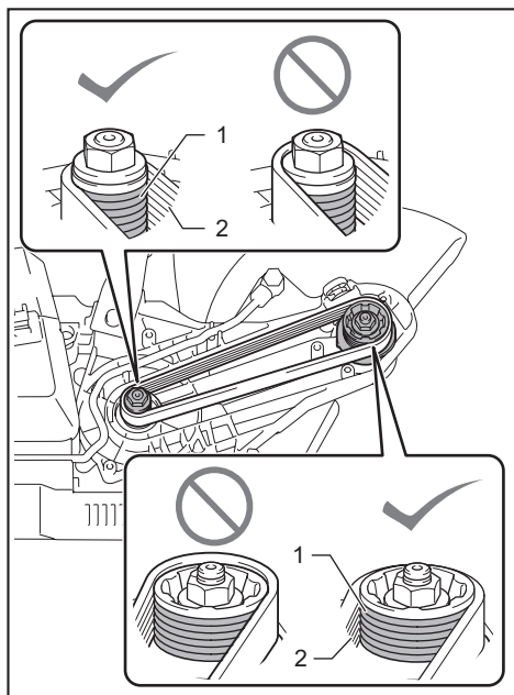
► 1. 皮帶輪上的導軌 2. 三角皮帶上的導件
