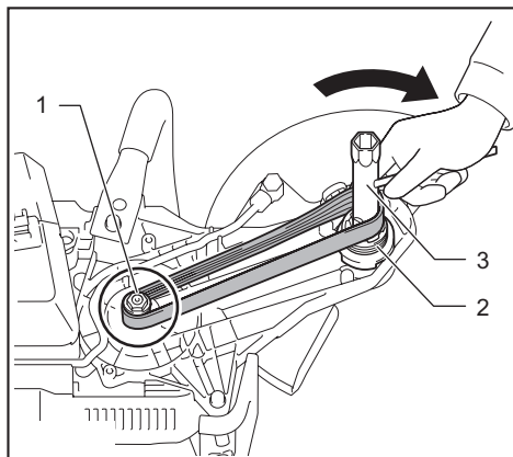
► 1. 皮帶輪（小） 2. 皮帶輪（大） 3. 套筒扳手
