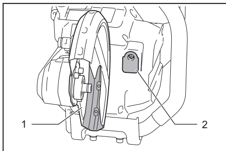
► 1. 砂輪罩 2. 燈具鏡片
