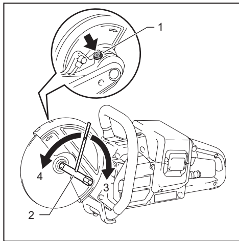
► 1. 軸鎖按鈕 2. 套筒扳手 3. 擰緊 4. 旋鬆
