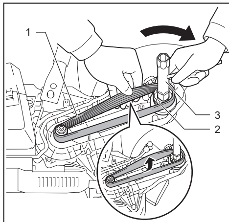
► 1. 三角皮帶 2. 皮帶輪（大） 3. 套筒扳手
