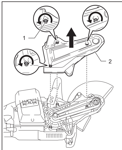
► 1. 六角套筒螺栓 2. 外蓋
