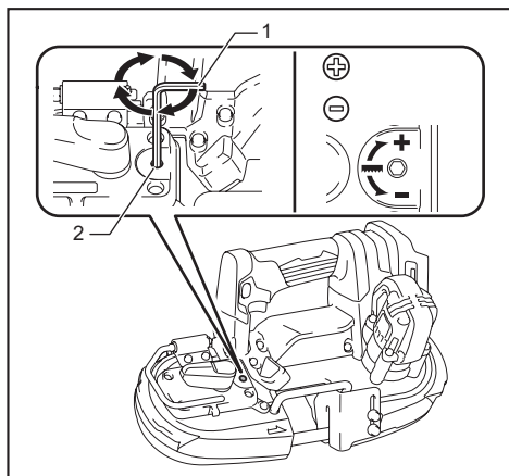
► 1. 六角扳手 2. 調整孔
