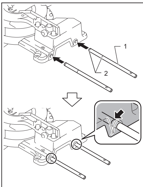
► 1. 桿件 2. 凹槽
