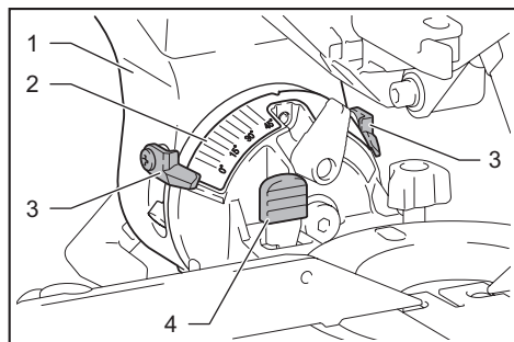
► 1. 支臂 2. 斜切刻度 3. 指針 4. 釋放桿的右側斜切角度
