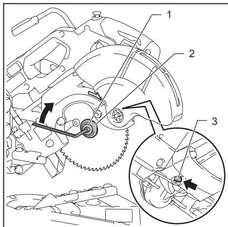
► 1. 六角套筒螺栓（左手側） 2. 外法蘭盤 3. 軸鎖
