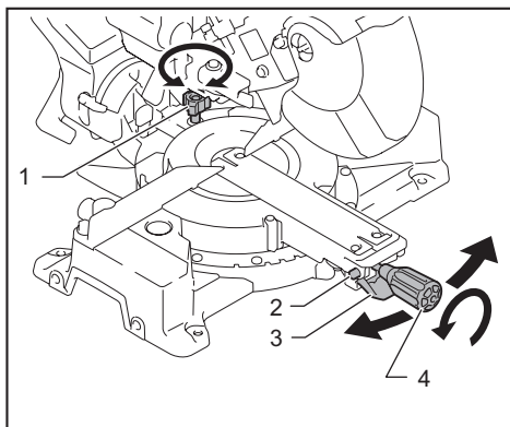
► 1. 調整旋鈕 2. 釋放鈕 3. 鎖定桿 4. 握把
