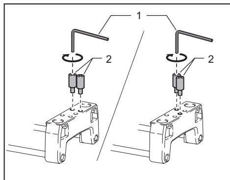
► 1. 六角扳手 2. 導板軸
