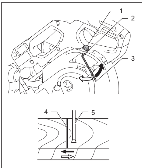
► 1. 調整螺絲 2. 範圍調整螺絲 3. 六角扳手 4. 雷射光線 5. 圓鋸機鋸片
