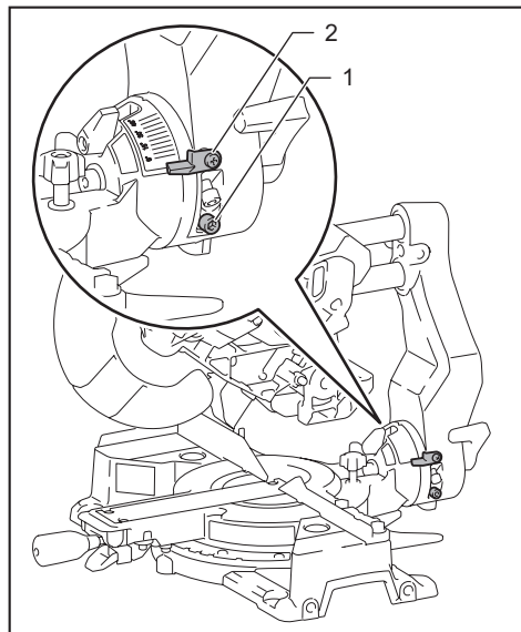
► 1. 0^\circ 調整螺栓 2. 指針上的螺絲
