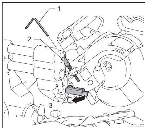
► 1. 六角扳手 2. 調整螺絲 3. 止動臂
