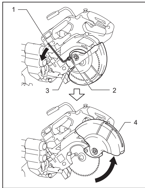
► 1. 六角扳手 2. 六角套筒螺栓 3. 中央蓋板 4. 鋸片保護罩
