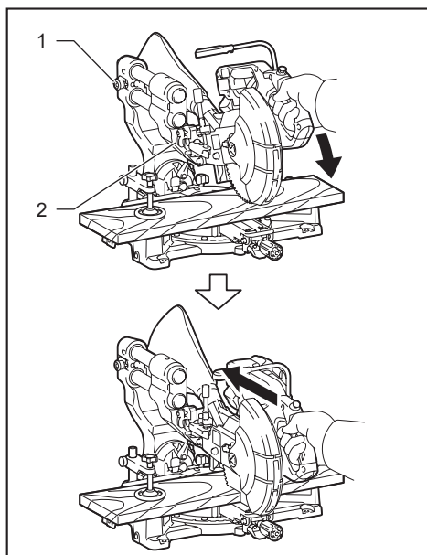
► 1. 止動銷 2. 擋桿
