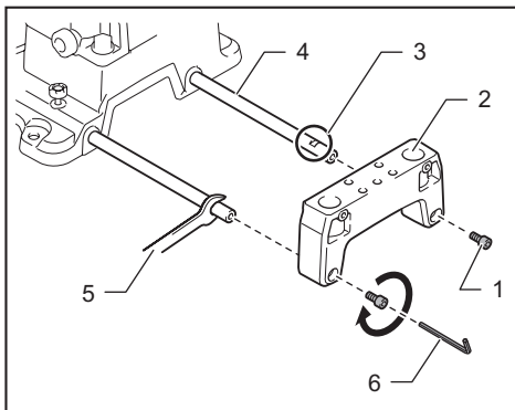
► 1. 六角套筒螺栓 2. 底基座 3. 平坦表面 4. 桿件 5. 扳手 6. 六角扳手
