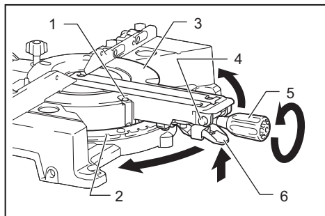
► 1. 指針 2. 斜接角度刻度 3. 旋轉基座 4. 釋放鈕 5. 握把 6. 鎖定桿
