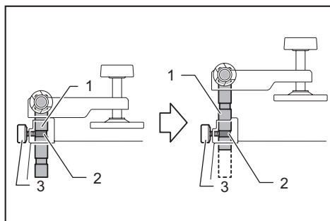
► 1. 虎鉗桿 2. 凹槽 3. 下部螺絲
