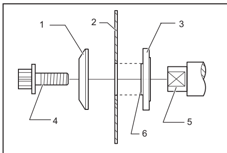
► 1. 外法蘭盤 2. 圓鋸機鋸片 3. 內法蘭盤 4. 六角套筒螺栓（左手側） 5. 心軸 6. 鋸片安裝部件
