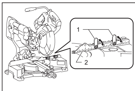
► 1. 小型副導板 2. 刻度
