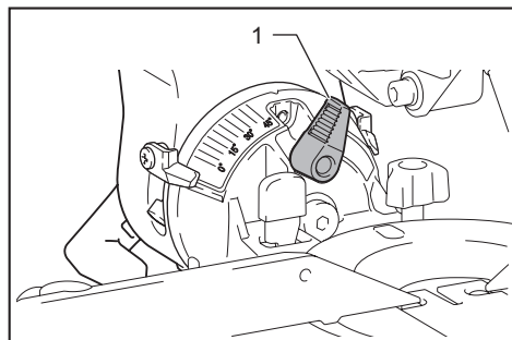
► 1. 釋放桿的 46^\circ 斜切角度
