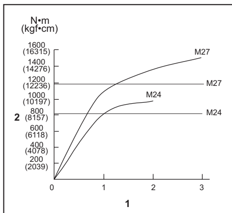
1. 緊固時間 (秒) 2. 扭力
