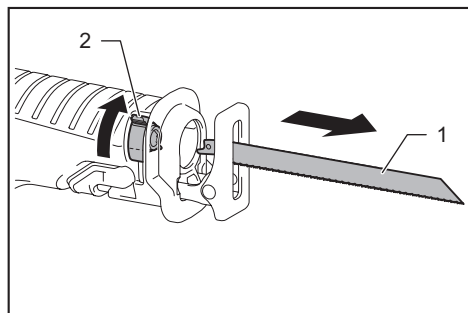
► 1. 手提鋸機鋸片 2. 釋放桿
