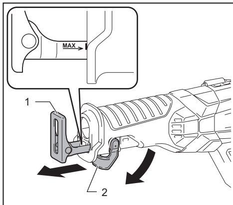
► 1. 軌座 2. 軌座調節杆
