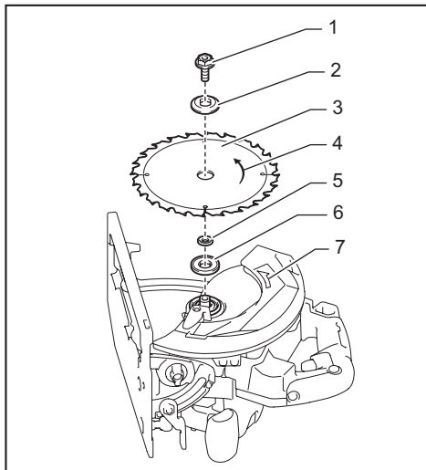
► 1. 六角螺栓 2. 外法蘭盤 3. 圓鋸機鋸片 4. 圓鋸機鋸片上的箭頭 5. 擋圈 6. 內法蘭盤 7. 工具上的箭頭
