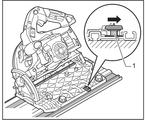
► 1. 滑桿
