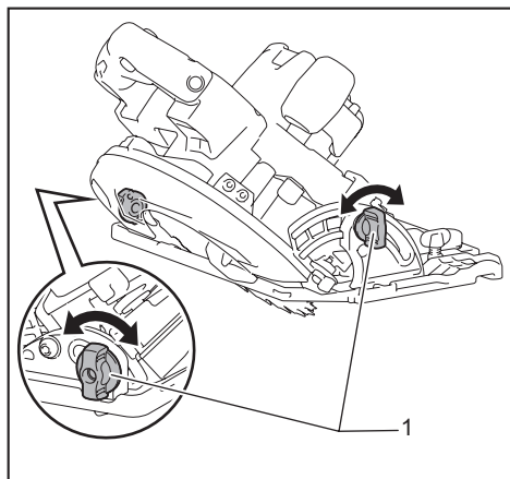
► 1. 夾緊螺絲
