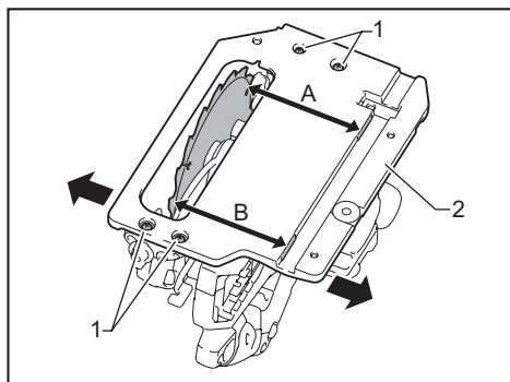
► 1. 螺絲 2. 基座
