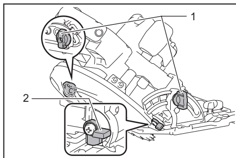
► 1. 夾緊螺絲 2. 止動器
