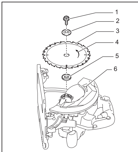
► 1. 六角螺栓 2. 外法蘭盤 3. 圓鋸機鋸片 4. 圓鋸機鋸片上的箭頭 5. 內法蘭盤 6. 工具上的箭頭
