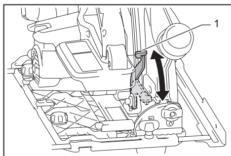
► 1. 桿
