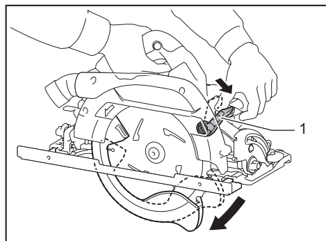
► 1. 縮回桿
