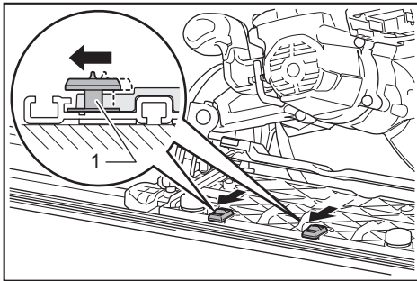
► 1. 滑桿
