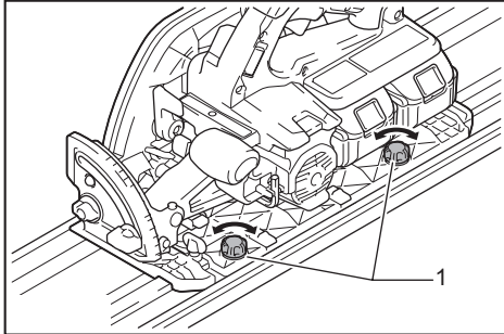
► 1. 調整螺絲
