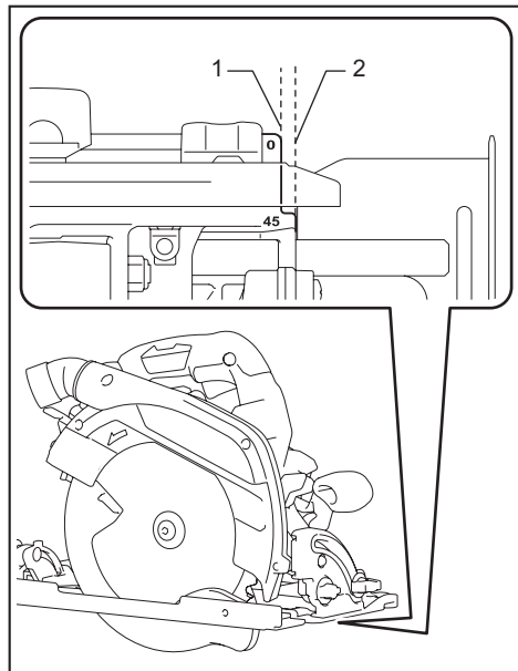
► 1. 切割線 (0° 位置) 2. 切割線 (45° 位置)
