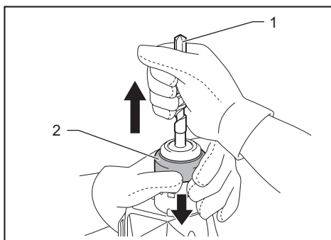
► 1. 鑽頭 2. 卡盤蓋
