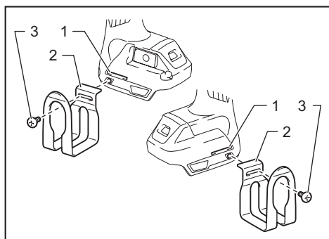
► 1. 溝槽 2. 鉤環 3. 螺絲
