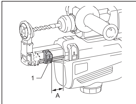
► 1. 深度調整按鈕
