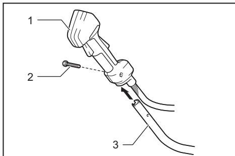
► 1. 握把 2. 螺絲 3. 把手桿
