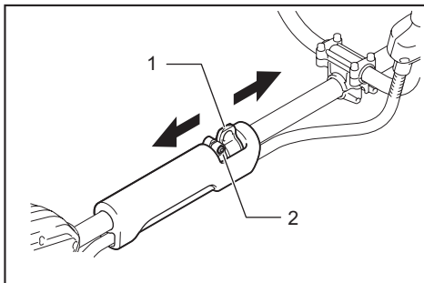
► 1. 吊扣 2. 內六角螺栓
