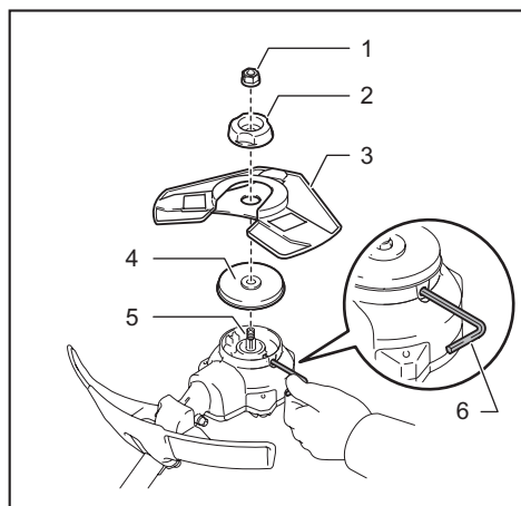
► 1. 螺帽 2. 夾緊墊圈 3. 刀頭刀片 4. 接收墊圈 5. 心軸 6. 六角扳手
