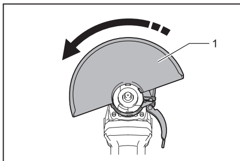
► 1. 砂轮罩
