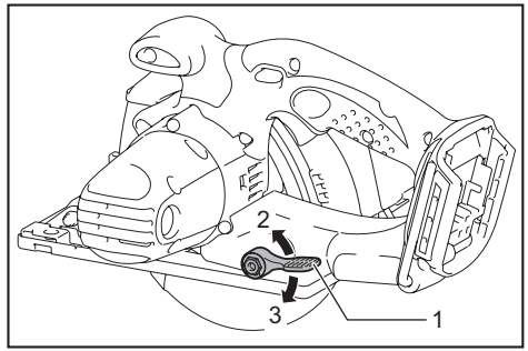
► 1. 杆 2. 拧松 3. 拧紧
