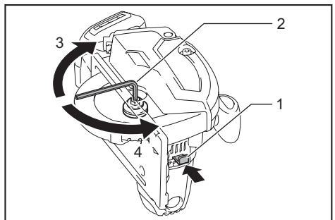
► 1. 轴锁 2. 六角扳手 3. 拧紧 4. 拧松
