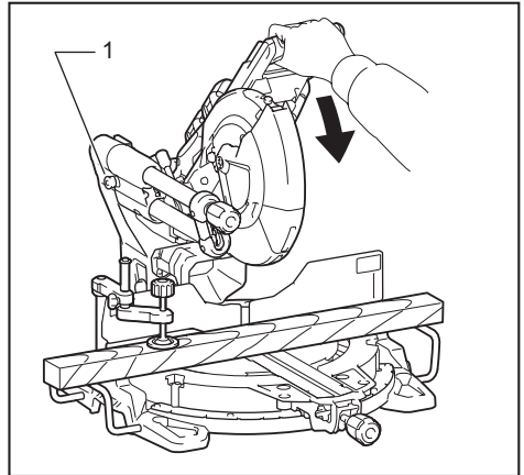
► 1. 止動銷
