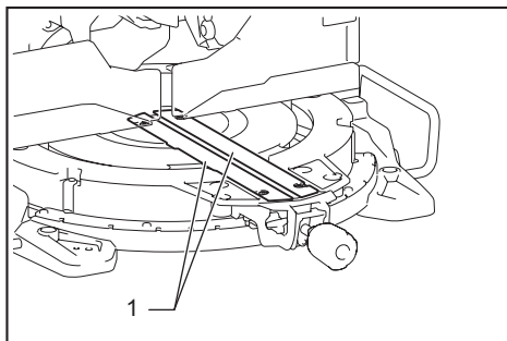
► 1. 鋸痕板
