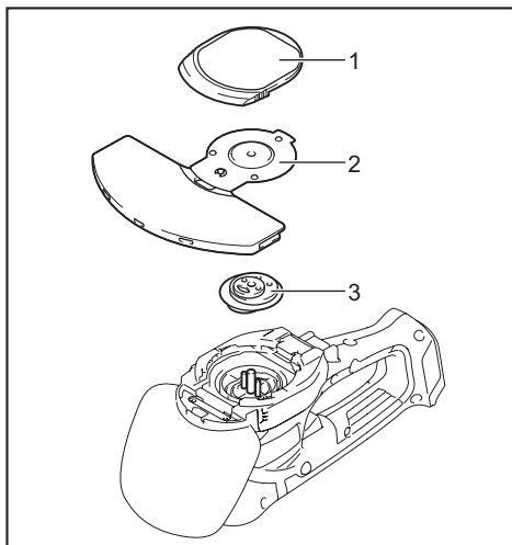
► 1. 底蓋 2. 刀片 3. 曲柄
