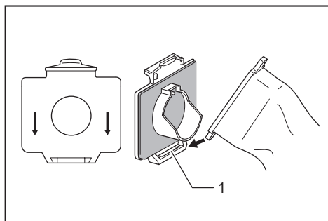
► 1. Lower groove
