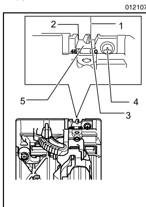
1. 切割线 2. 45^\circ 位置 3. 0^\circ 位置 4. 螺丝 5. 顶部导板
