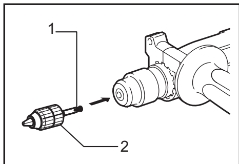
► 1. 卡盘适配器 2. 手紧式钻机卡盘
