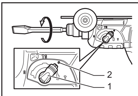
► 1. 动作模式变换钮 2. O 符号
