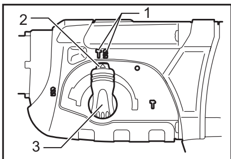
► 1. 旋转并冲击 2. 锁定按钮 3. 动作模式变换钮
