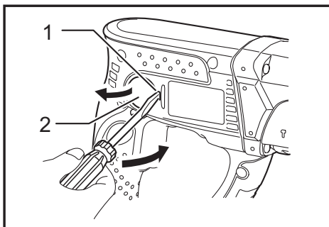
► 1. 凹槽部分 2. 夹盖
