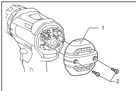
1. 后盖 2. 螺丝
