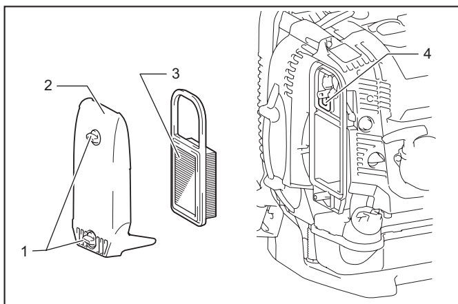
► 1. 旋钮螺栓 2. 空气过滤器盖 3. 组件 4. 通气阀
