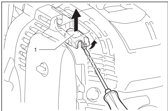
► 1. 化油器盖
