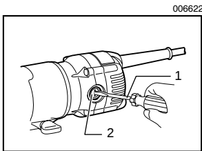
1. 螺丝起子 2. 碳刷盖
