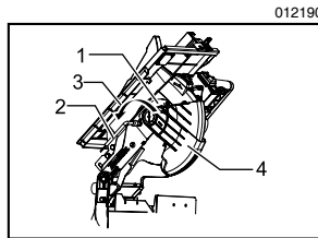
1. 中心盖板 2. 套筒扳手 3. 六角螺栓 4. 下部锯片保护罩 A
