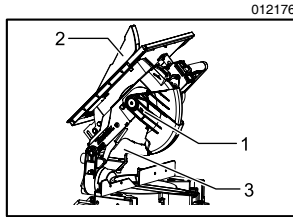
1. 下部锯片保护罩 A 2. 上部锯片保护罩 3. 下部锯片保护罩 B
