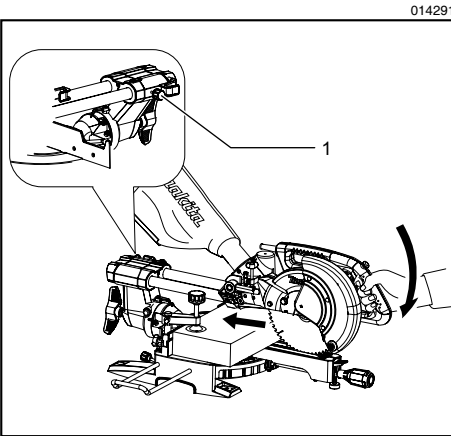
1. 锁定螺丝
